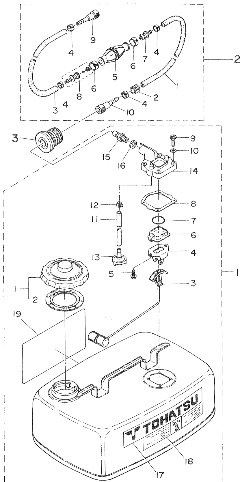
オプションパーツ (Ⅲ) アクセサリー (3) オートエアベント Fig. 26-A OPTIONAL PARTS (III) ACCESSORIES (3) AUTO AIR VENT
