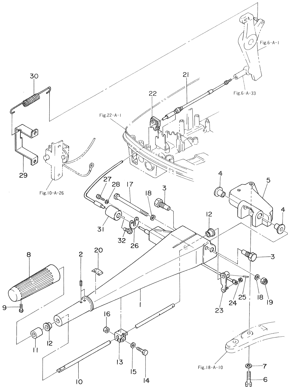
Fig. 7-A バーハンドル (EFT/EF) BAR HANDLE (EFT/EF)
