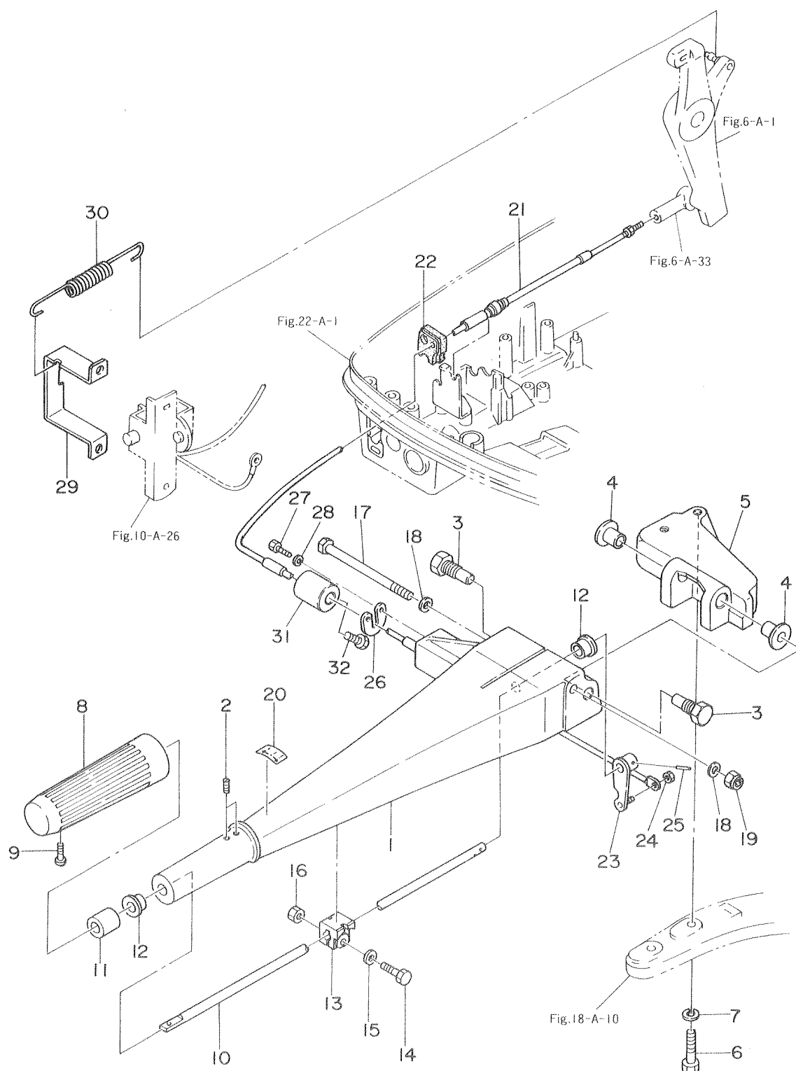
バーハンドル (EFT/EF) Fig. 7-A BAR HANDLE (EFT/EF)
